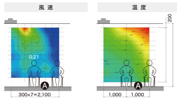
CASE 2 (200CMH) 吹出温度: 18°C、室内温度: 28°C
