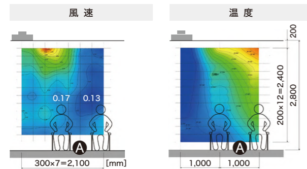
CASE 1 (300CMH) 吹出温度: 18°C、室内温度: 28°C
